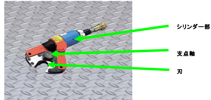
写真1：油圧電線カッター
